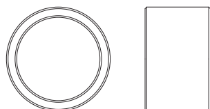
13. Spacer, 25.5 ID x 31.8 OD x 20 QTY 2
