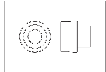
24. Bushing, guide rod retainer QTY 2
